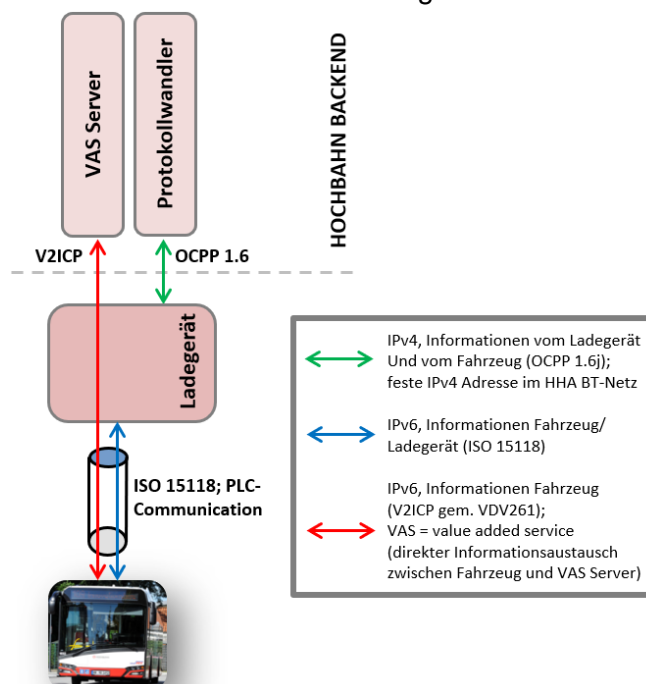
Abbildung 3: Kommunikationskonzept
